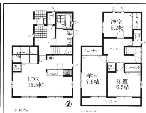
1号棟 平面図
