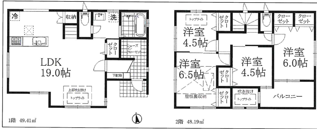
2号棟 平面図
